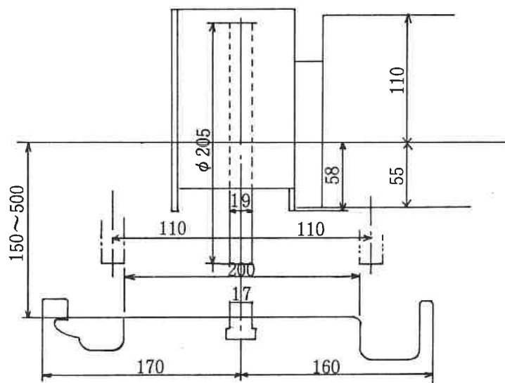
加工範囲図
