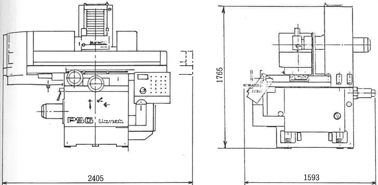
外形図
