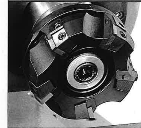
標準カッター〔スローアウェイトップ サイズ=15.875mm〕
